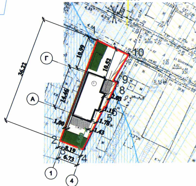
Разбивочный чертеж. М 1:500
