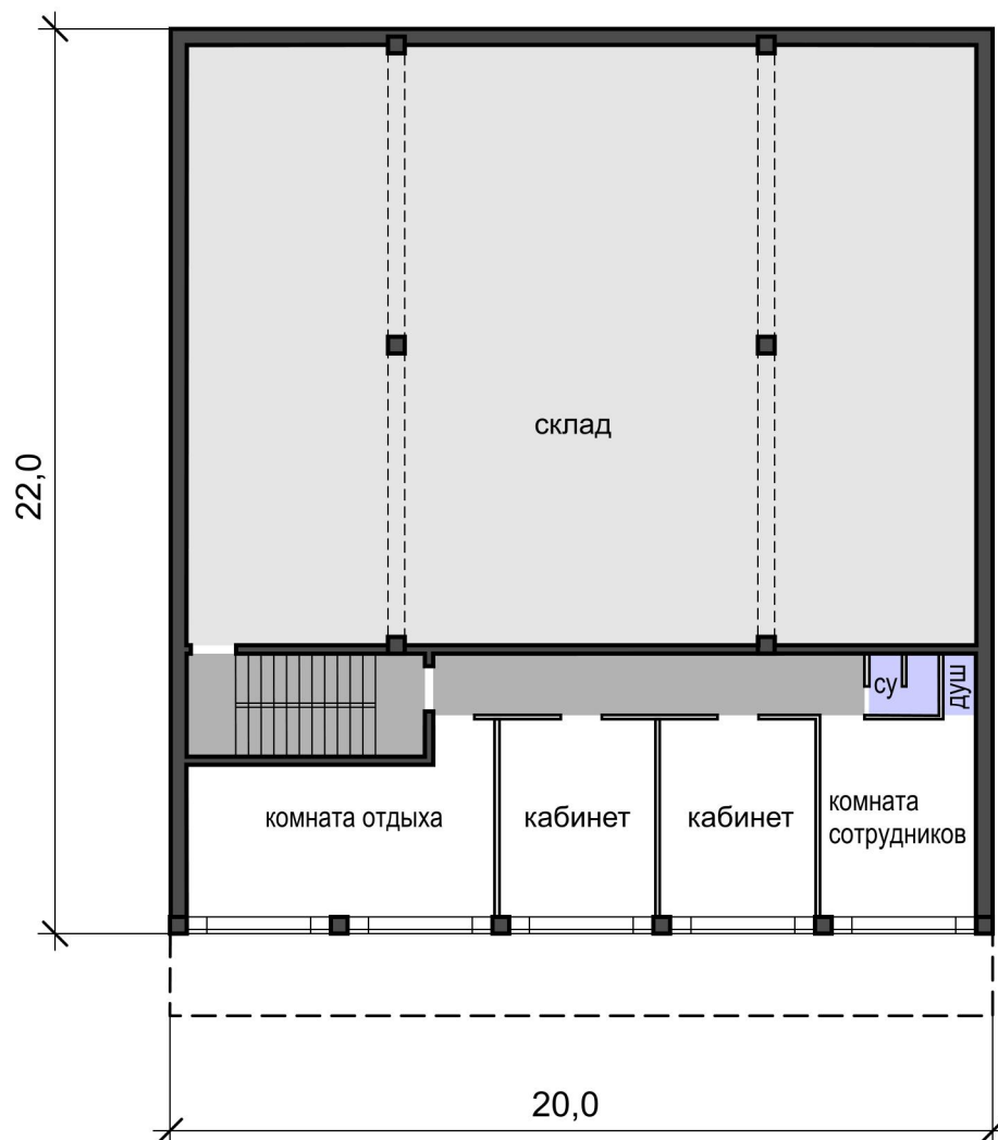
2-й этаж
