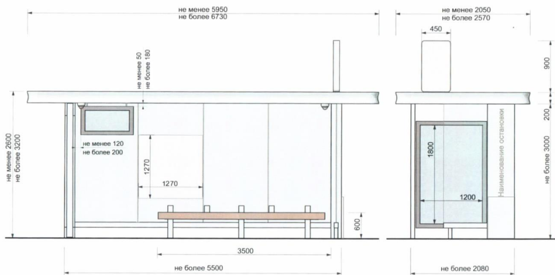
Основные габаритные размеры остановочного павильона - не менее 5950 x 2600 x 2050 и не более 6730 x 3200 x 2570 мм.
