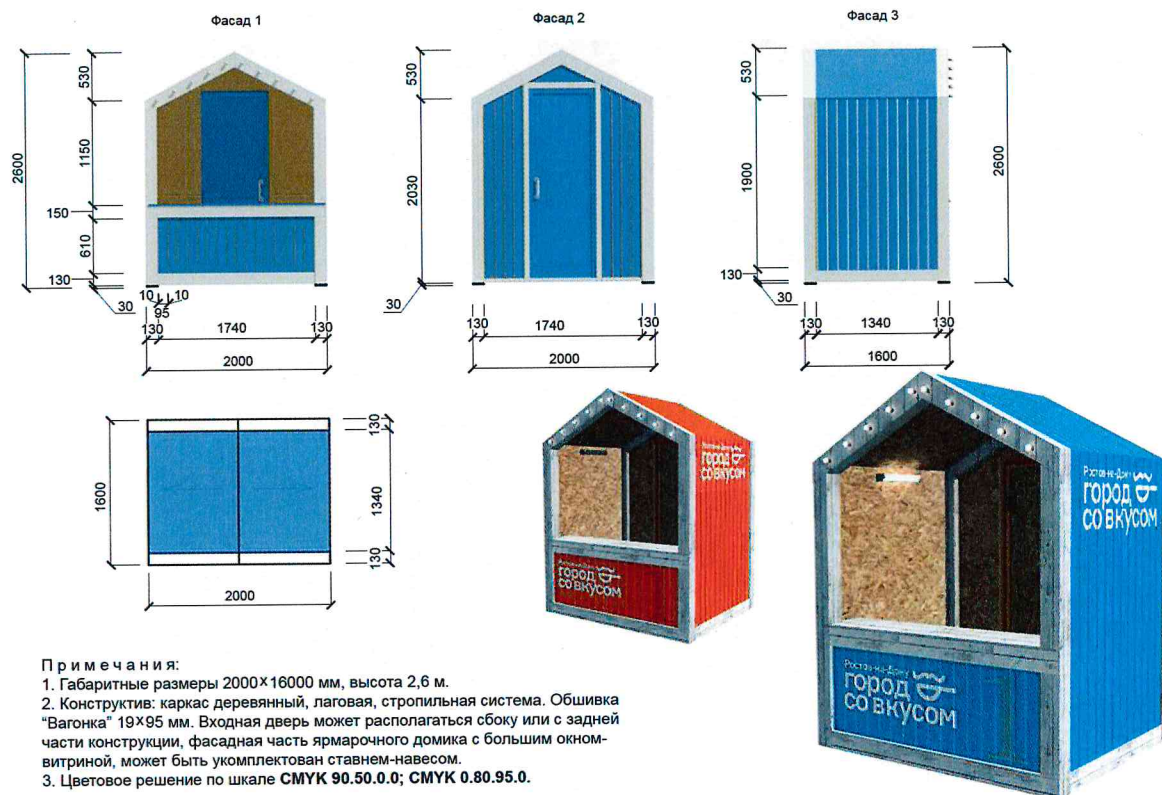
Рисунок А.8 — Ярмарочный домик 2×1,6 м
