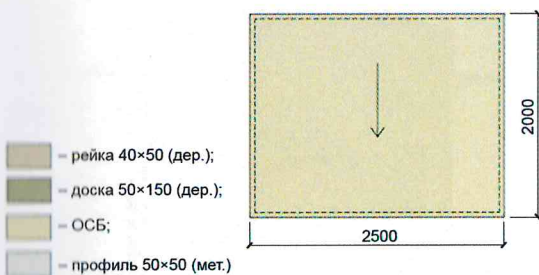
Рисунок А.7 — Павильон 2,5×2 м, тип 3
