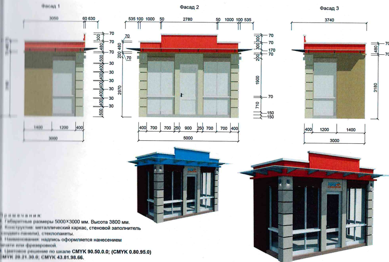
Рисунок А.10 — Павильон 5×3 м
