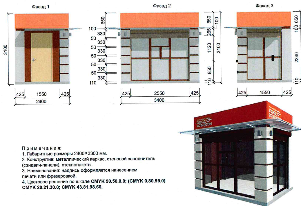
Рисунок А.9 — Киоск 3,4×2,4 м
